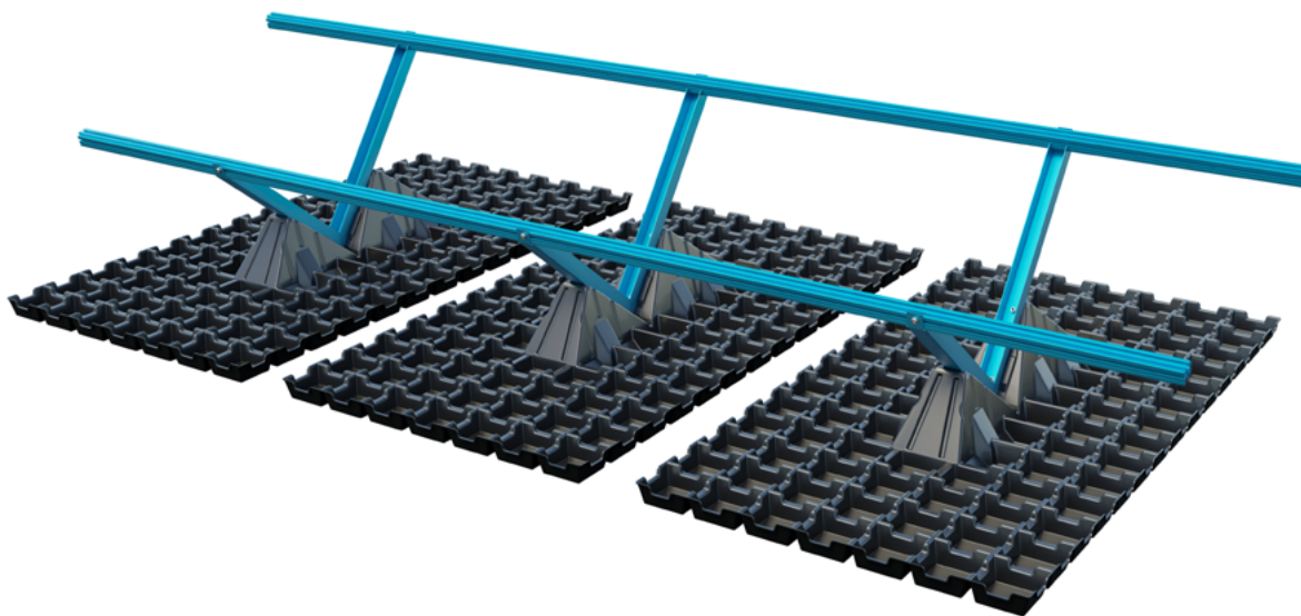
Abbildung: Fertige Montage der Systemträgerlage.
