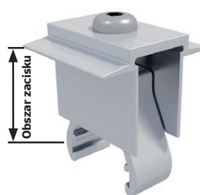
Uchwyt modułu (MH)
